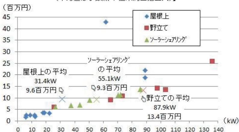
【図K・中小規模グループにおける2019年度以降の発電所施工費と出力数の分布（平均値は小数点1位未満四捨五入）】
