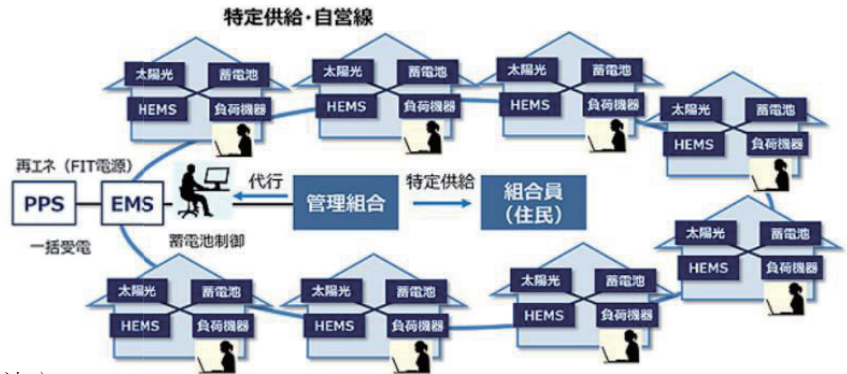
▲マイクログリッドシステムの構成
