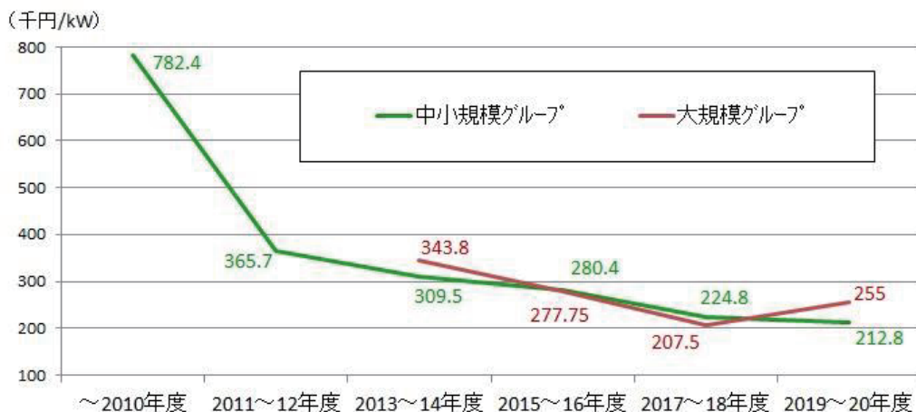
【図 C・平均施工費単価の推移（数字は千円/kW、ただしkWはモジュール出力）】
