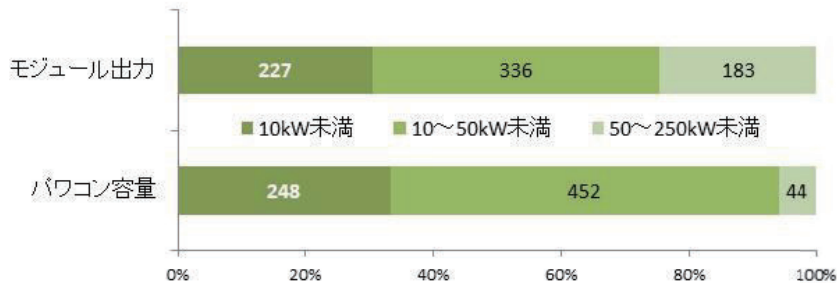
【図M・中小規模グループにおけるモジュール出力と パワコン容量（グラフ内数字は発電所数）】
