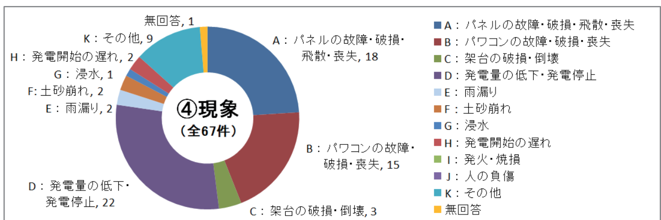
【図表ア・市民太陽光発電所のトラブル分類(単位：件)】
